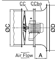
Esempi di installazione Installation example
